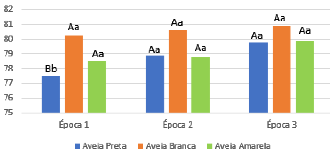
Figura 4: Percentagem de folhas das espécies de aveia nas épocas de semeadura. Letras maiúsculas representam diferença estatística entre as épocas e letras minúsculas dentro da época de semeadura.
