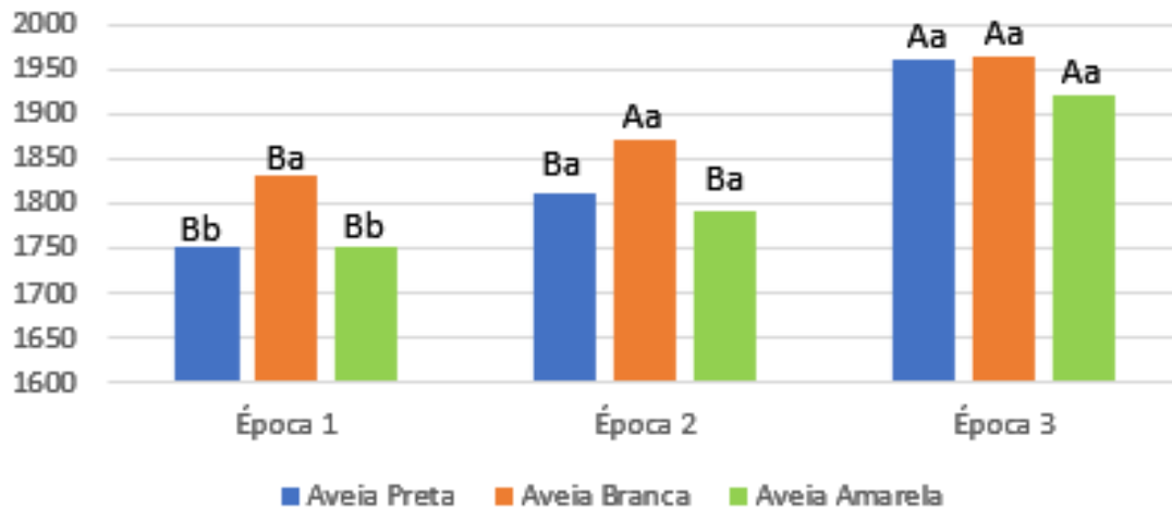
Figura 5: Produtividade de grãos das espécies de aveia nas épocas de semeadura. Letras maiúsculas representam diferença estatística entre as épocas e letras minúsculas dentro da época de semeadura.
