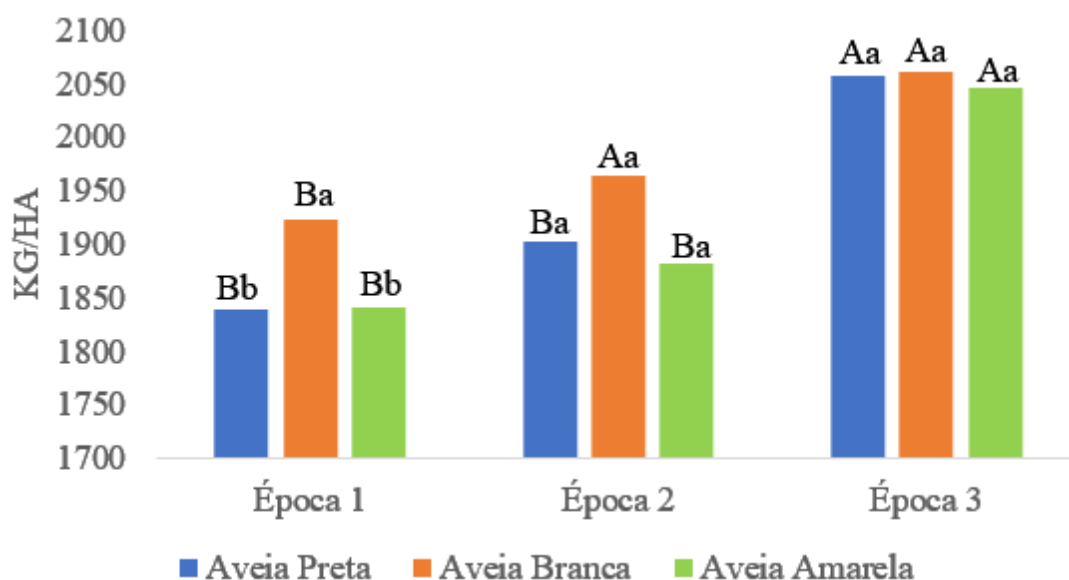
Figura 3: Matéria seca das espécies de aveia nas épocas de semeadura. Letras maiúsculas representam diferença estatística entre as épocas e letras minúsculas dentro da época de semeadura.
